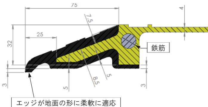
A-A断面
